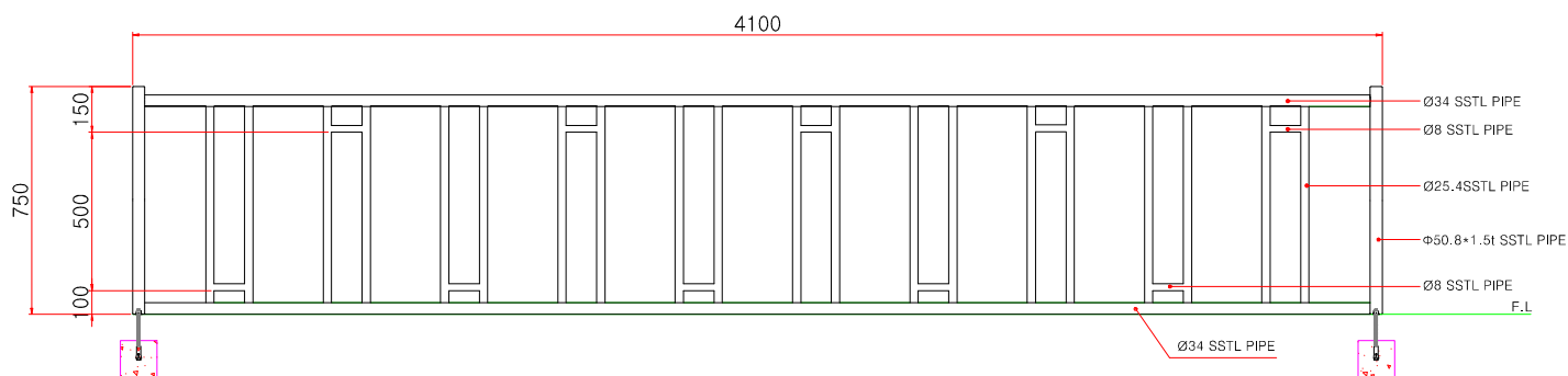
정면도
