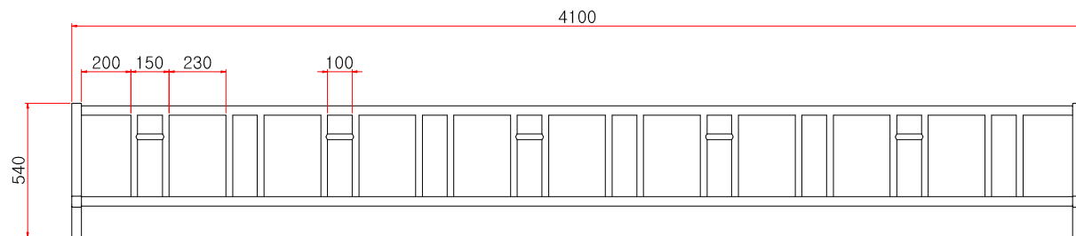
평면도
