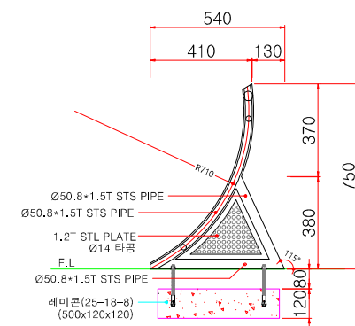
측면도
